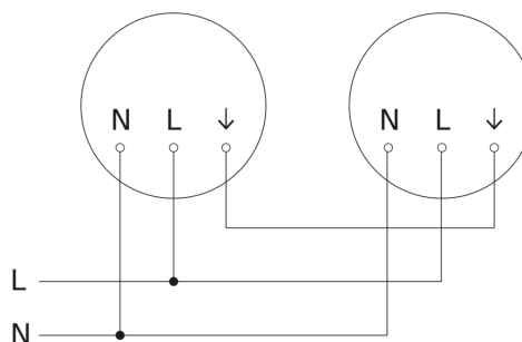
aansluitschema master/master
